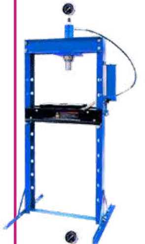
BWR5118 Υδραυλική πρέσα • Με αντλία χείρος • 12Ton • Διαδρομή εμβόλου 175mm
