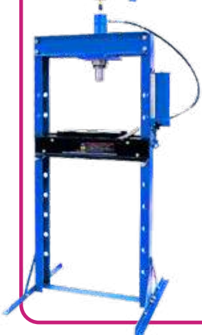
BWR5230 Υδραυλική πρέσα • Με αντλία χείρος • 20Ton • Διαδρομή εμβόλου 185mm
